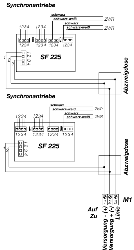
Synchronantriebe mit Zusatzverriegelung und externer Synchron-Folgesteuerung SF 225
