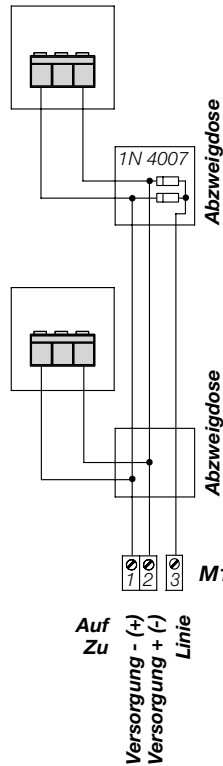
Kettenantrieb SKA 45, 50
