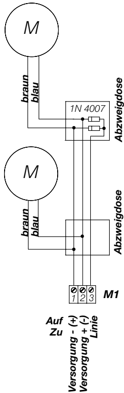
Spindeltrieb SA
